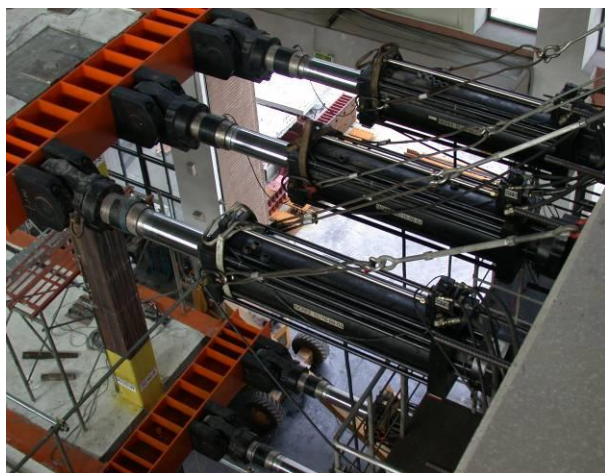
圖八 靜態油壓致動器
